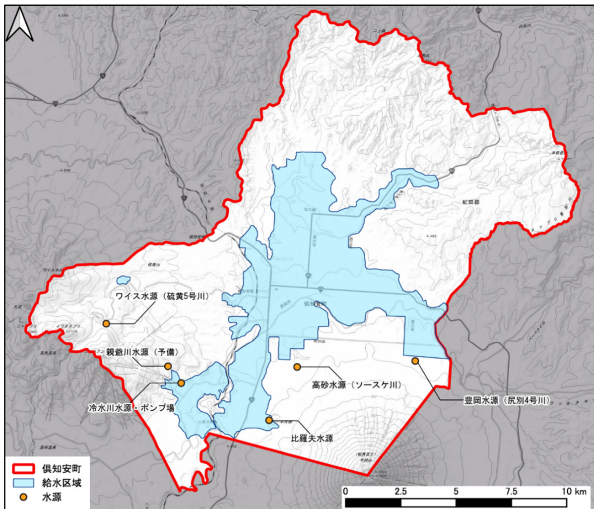
図 2-18 倶知安町の水道施設位置図
