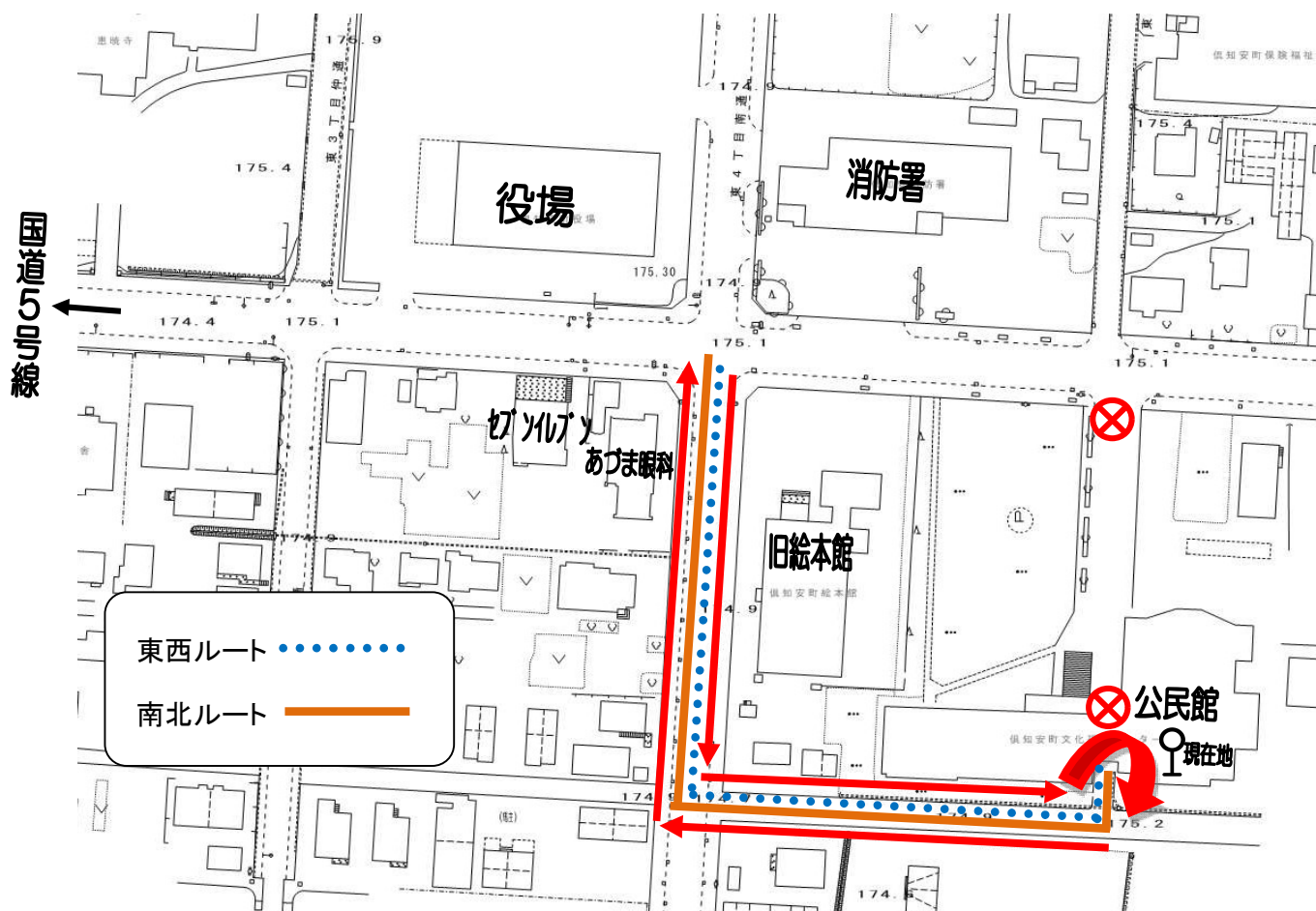
【変更位置図】
