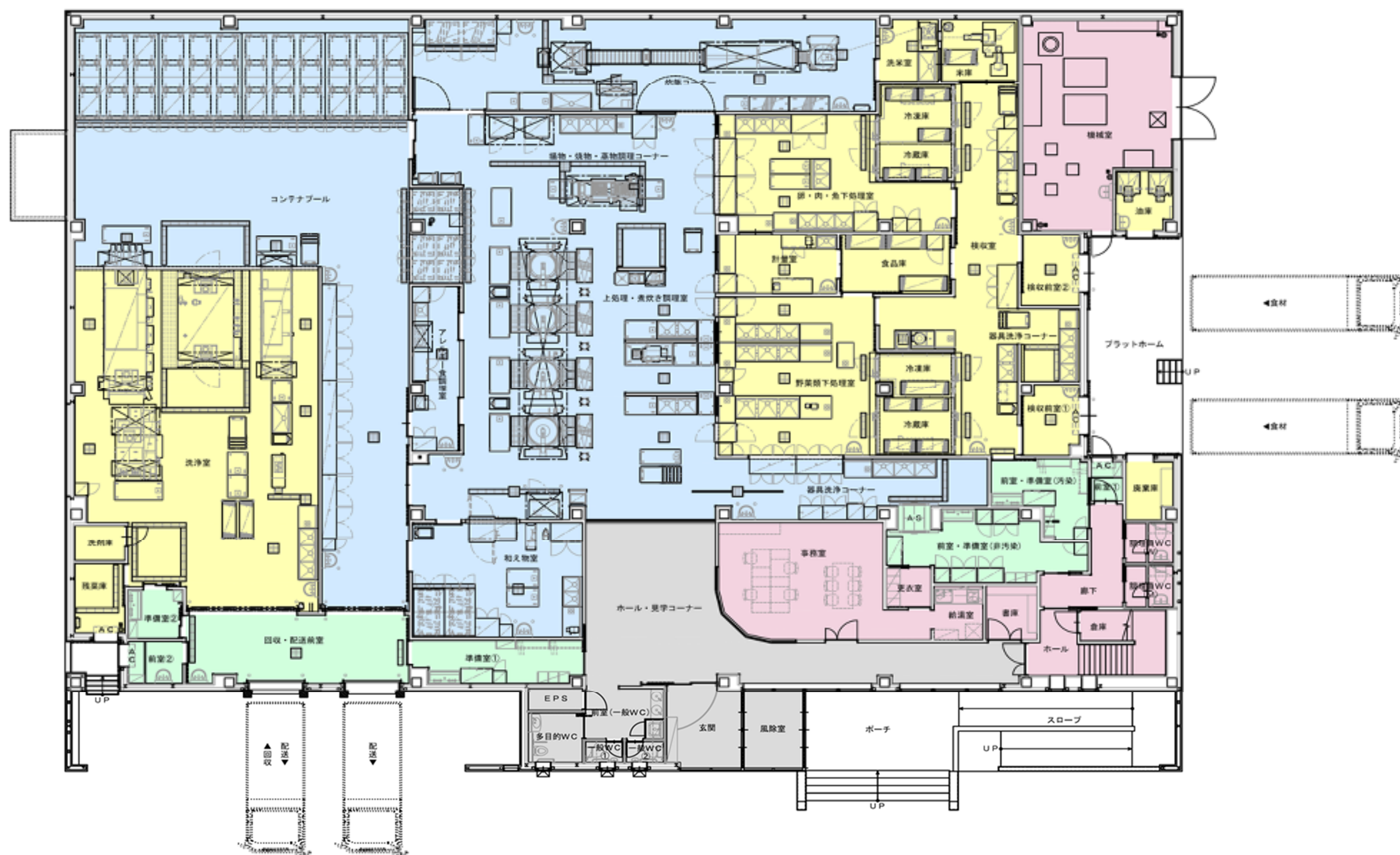
俱知安町学校給食センター 1F平面図
