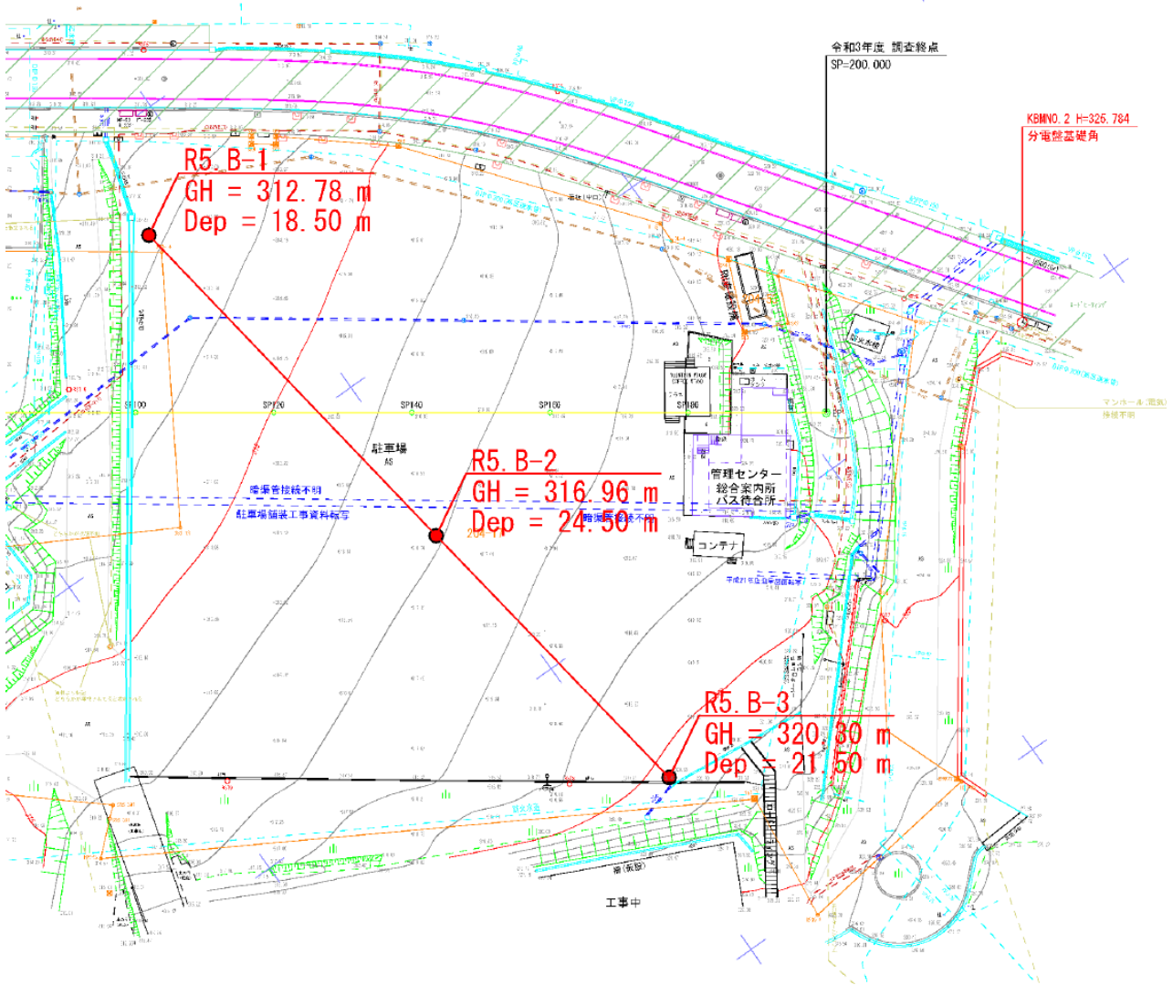
図 - 1.2 調査位置平面図 (S=1:1,000)
