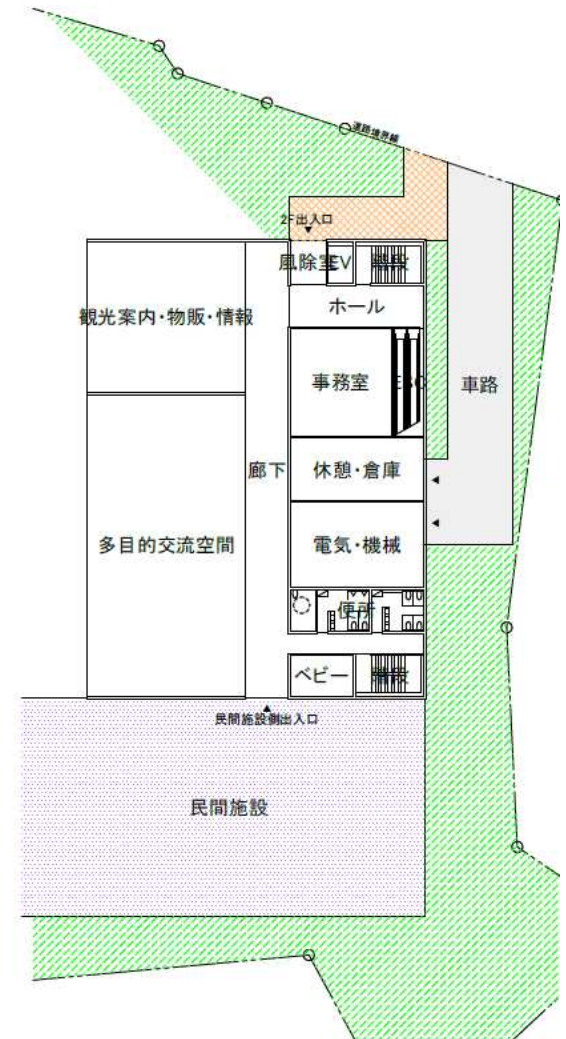
2階平面図
