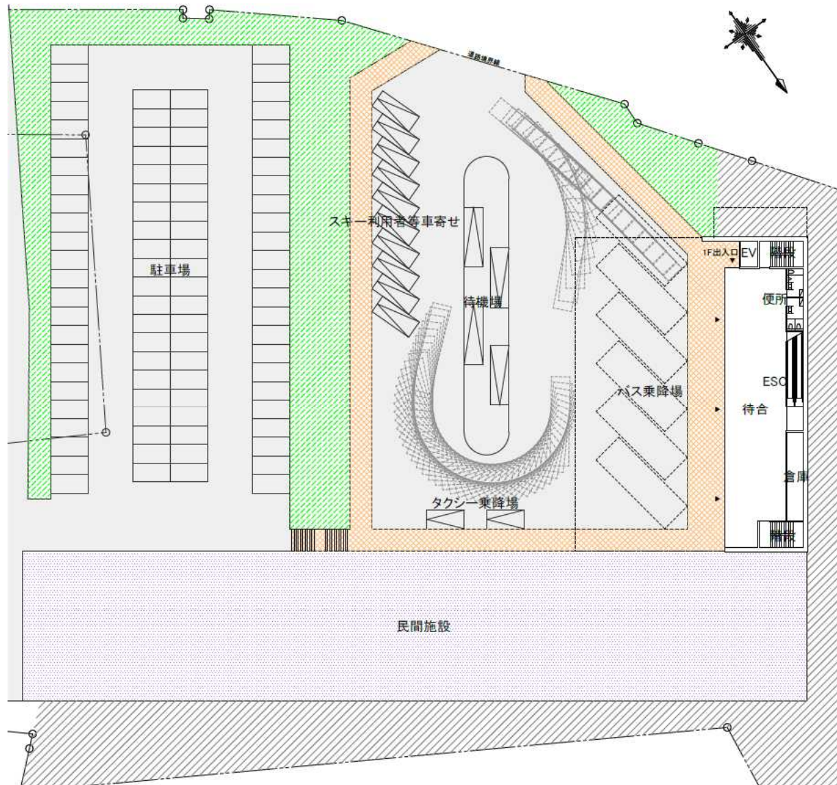
配置図兼1階平面図
