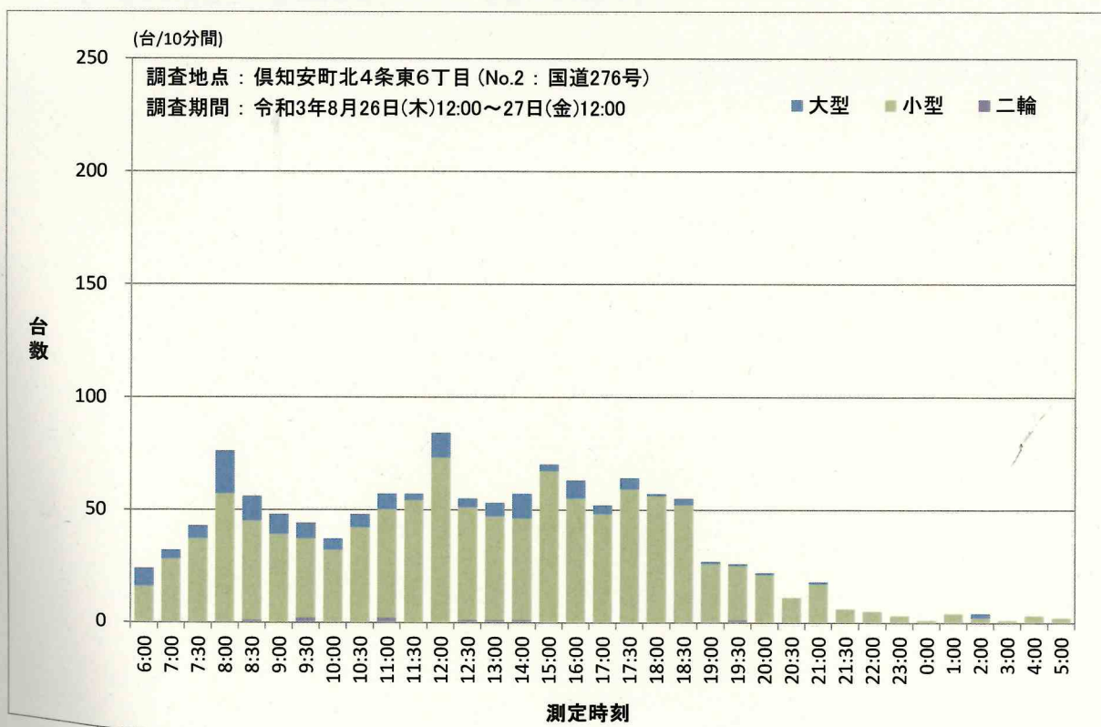
図 3-2 No. 2 地点：国道 276 交通量調査結果 (10 分値)
